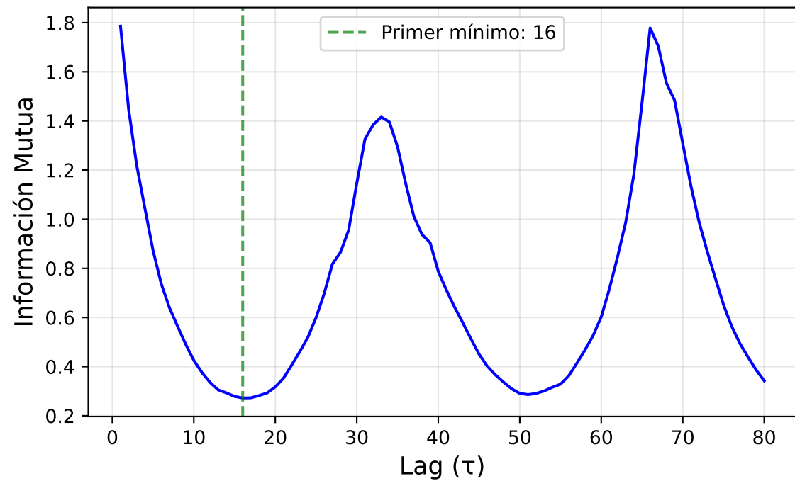
Información Mutua
