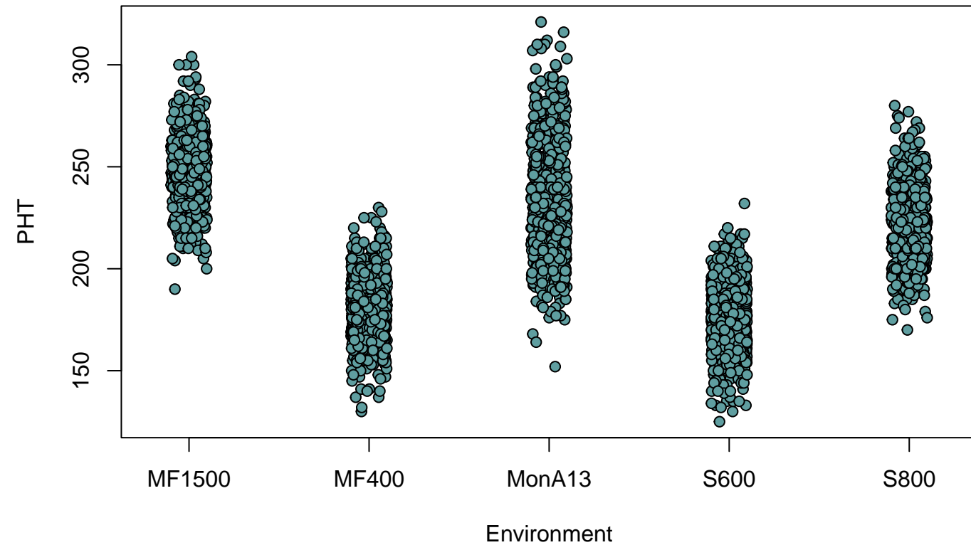
Stripchart of raw PHT values
