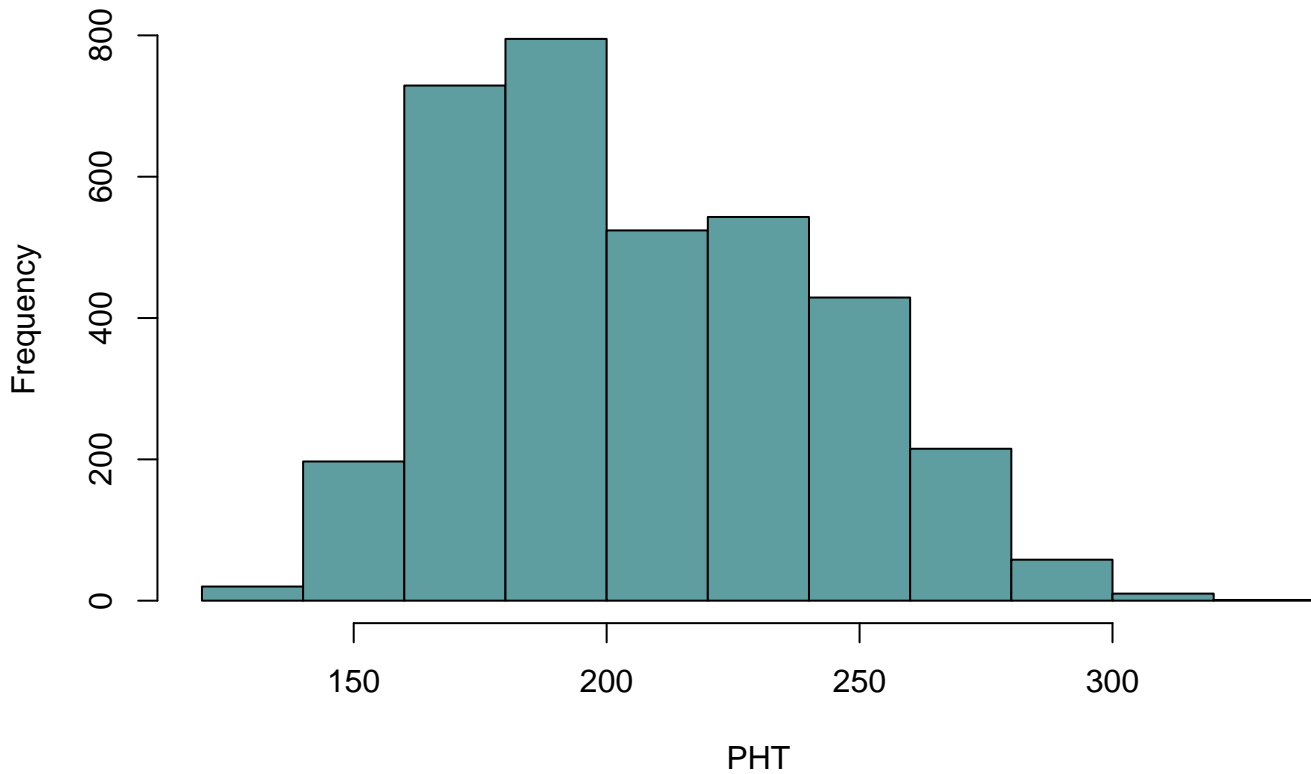
Histogram of raw PHT values
