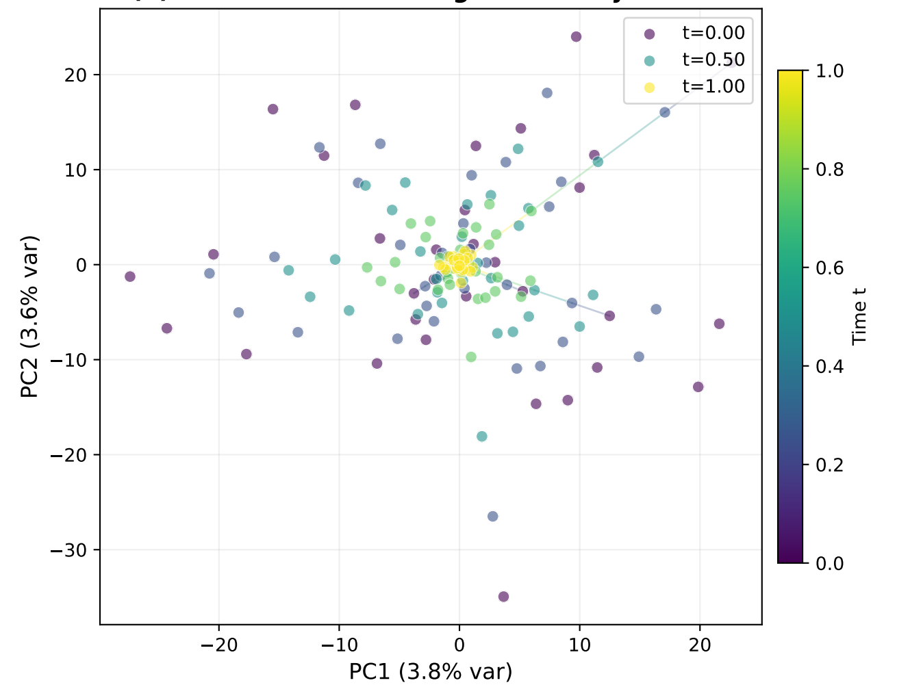
(d) PCA of Flow Matching Latent Trajectories
