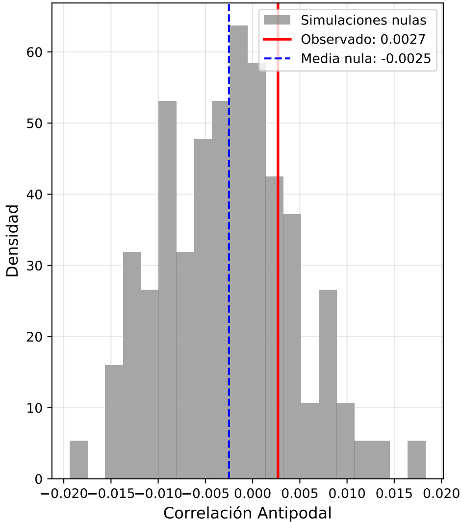
Test de Hipótesis Nula Z=0.74 , p=0.4568
