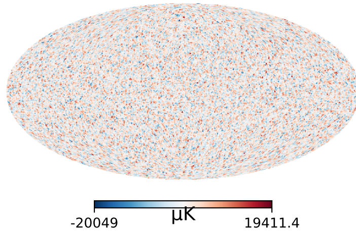
CMB Map (Simulación con Cl Planck 2018)
