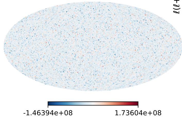
Correlación Antipodal Local T(\hat{n}) \cdot T(-\hat{n})
