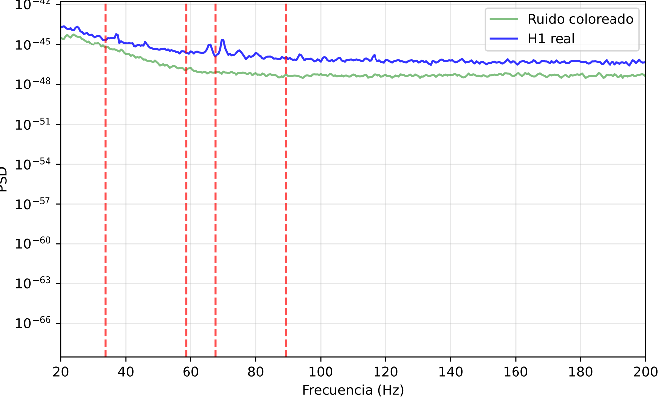
PSD: Ruido Coloreado vs LIGO Real
