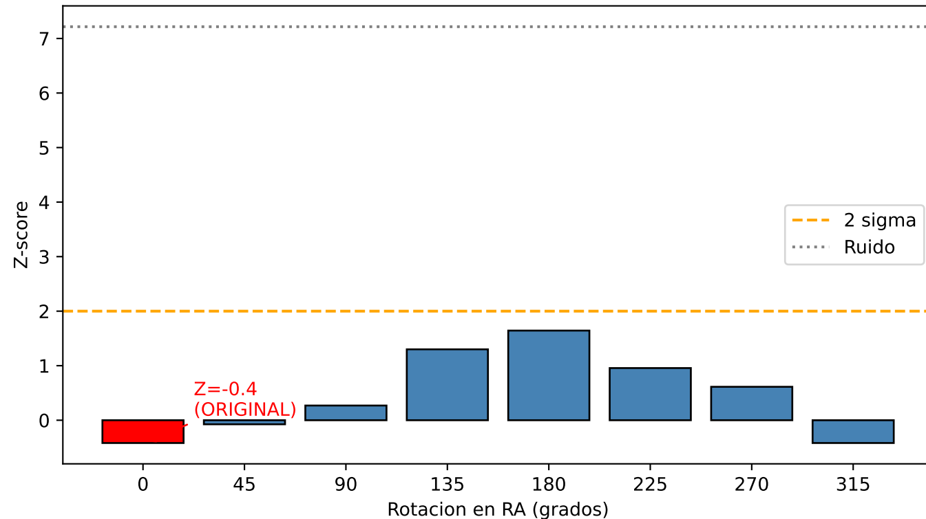
Correlacion CMB-LIGO vs Rotacion
