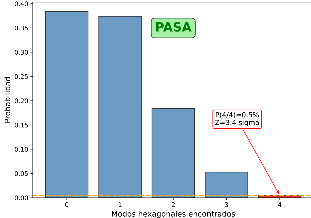
SANITY CHECK #1: Test Placebo (1000 realizaciones de ruido puro)
