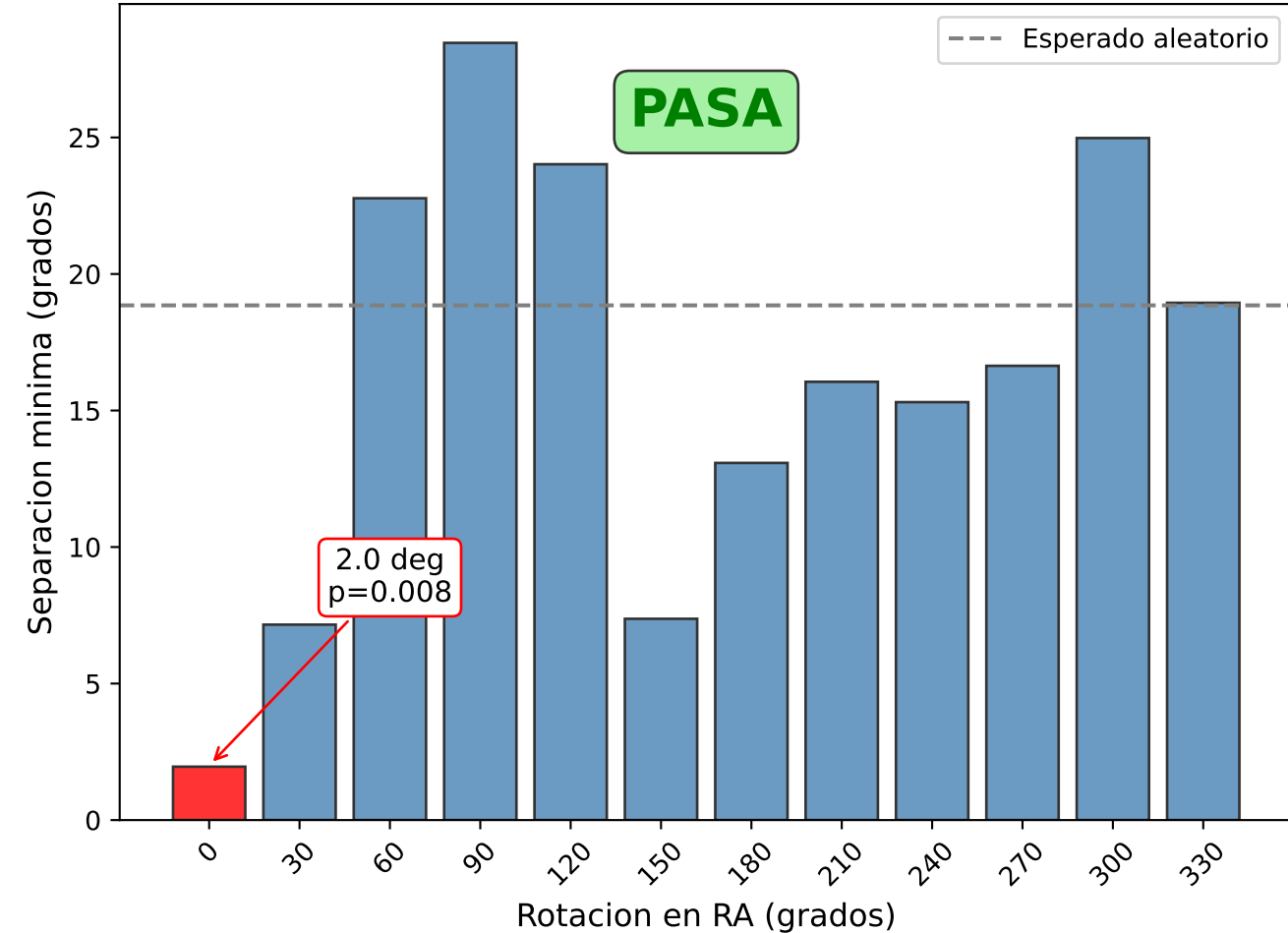
SANITY CHECK #2: Test de Rotacion (GW190814 - Polo Sur Galactico)
