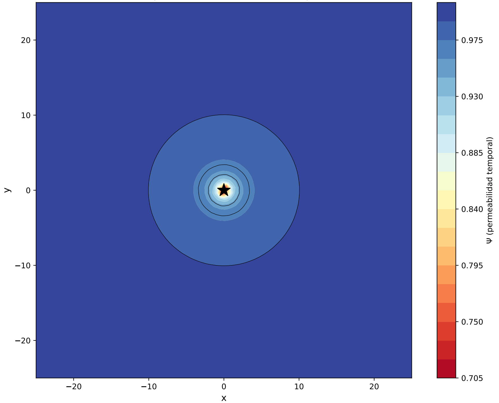
Campo \Psi = \sqrt{1 - r_s/r} Tiempo LENTO cerca de masa (rojo)
