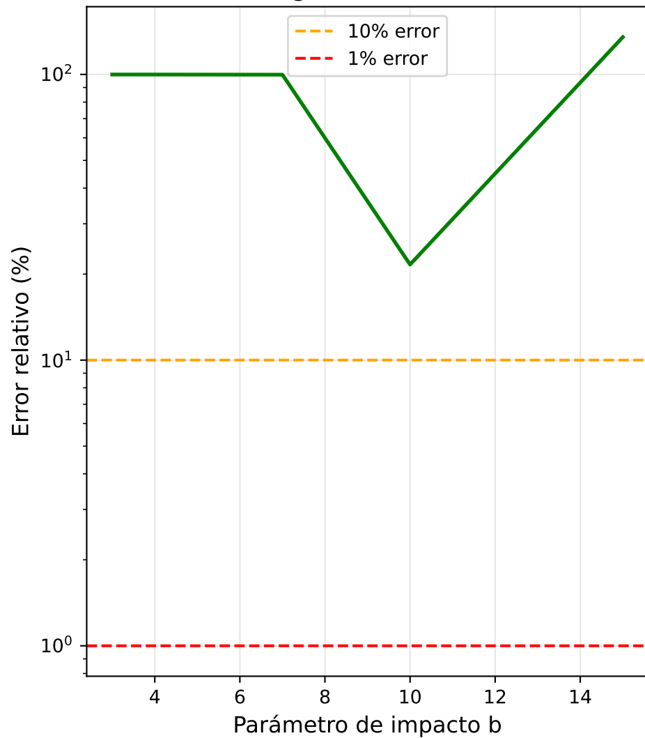
Convergencia OCTH \rightarrow GR
