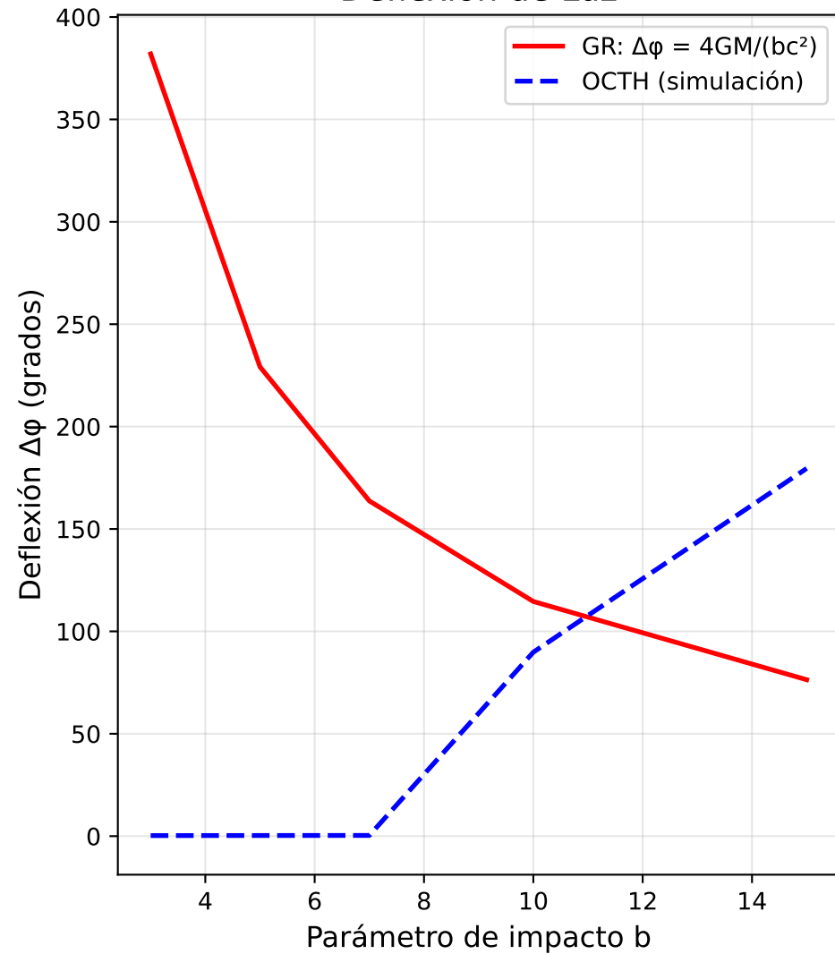
Deflexión de Luz
