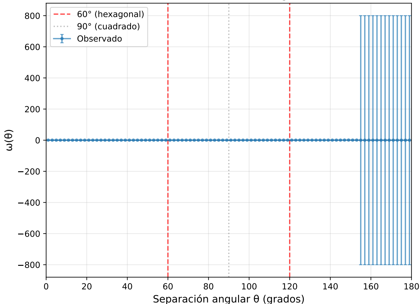
Función de Correlación Angular
