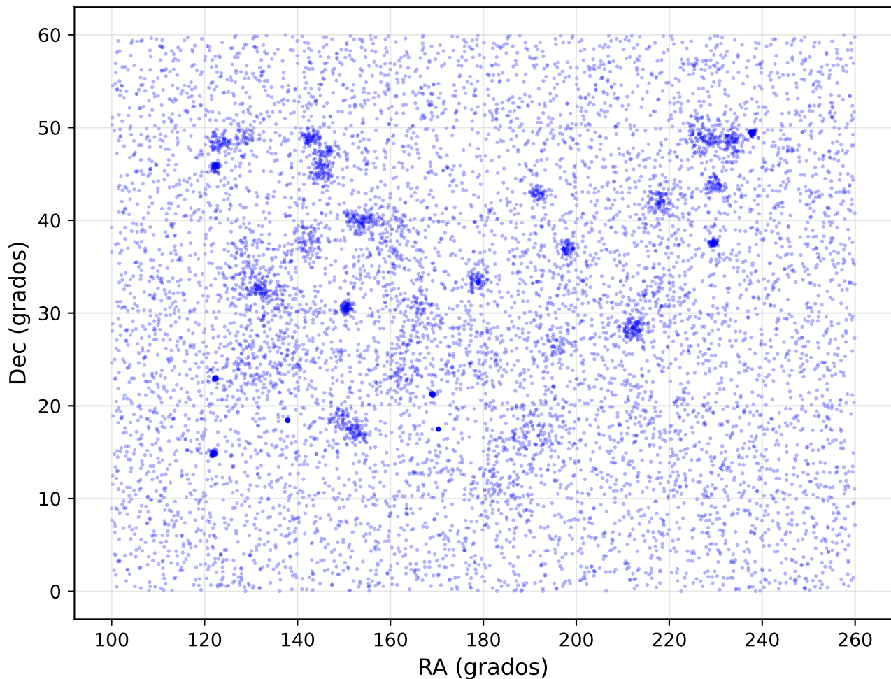
Comparación Hexagonal vs Control Exceso: 0.0215, Z=1.85
