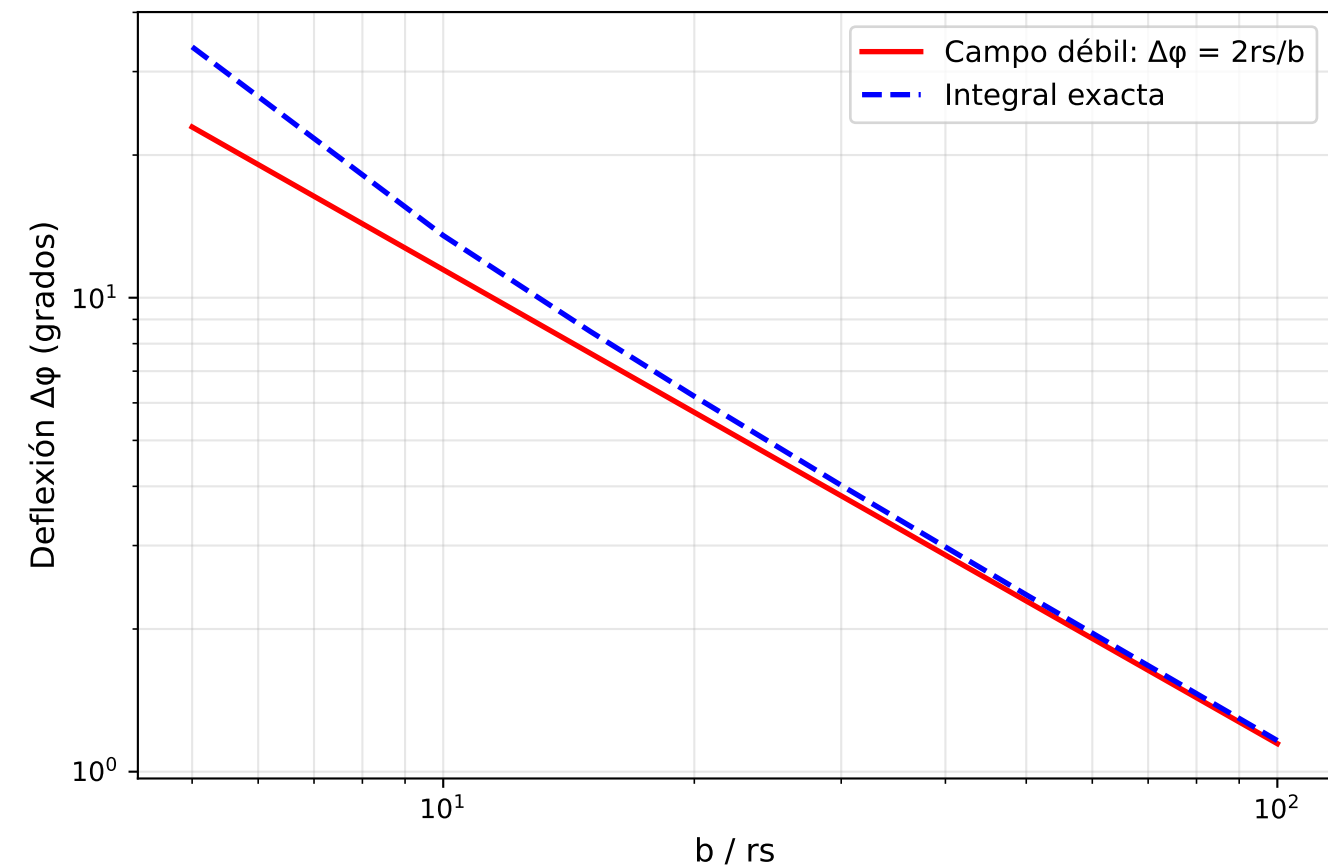
Deflexión de Luz en Métrica OCTH
