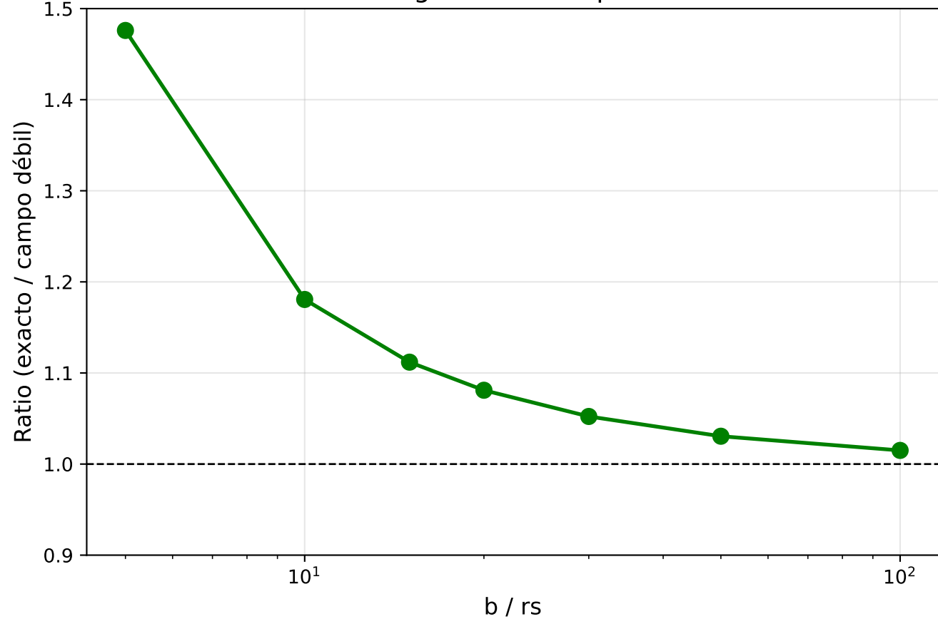
Convergencia a Campo Débil
