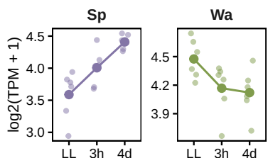
G APX6 ( p = 6.4e-04 )
