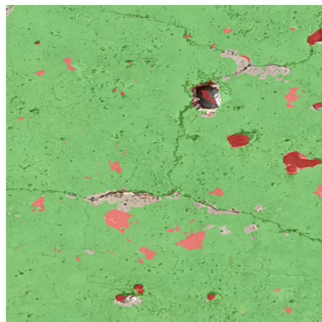
SegFormer
