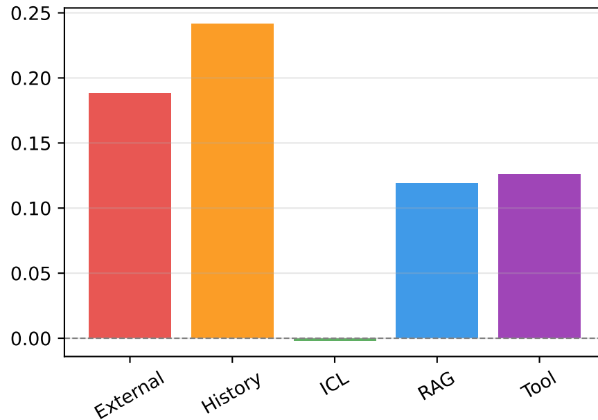
Mean Disc_{\Delta}
