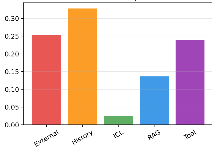
Mean UAI_{pls}
