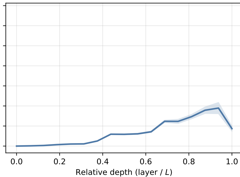
Llama 1B (16L)
