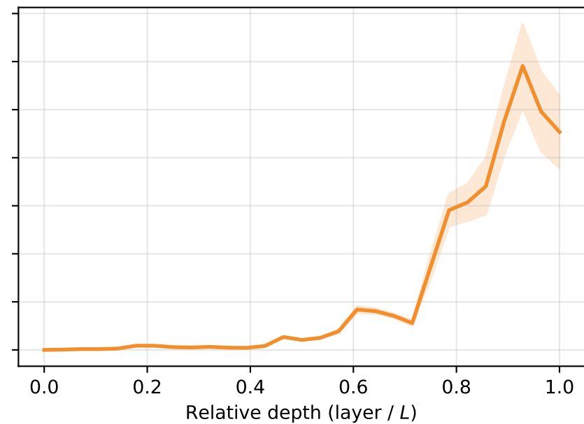
Llama 3B (28L)
