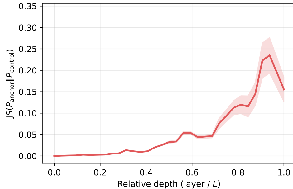
Llama 8B (32L)
