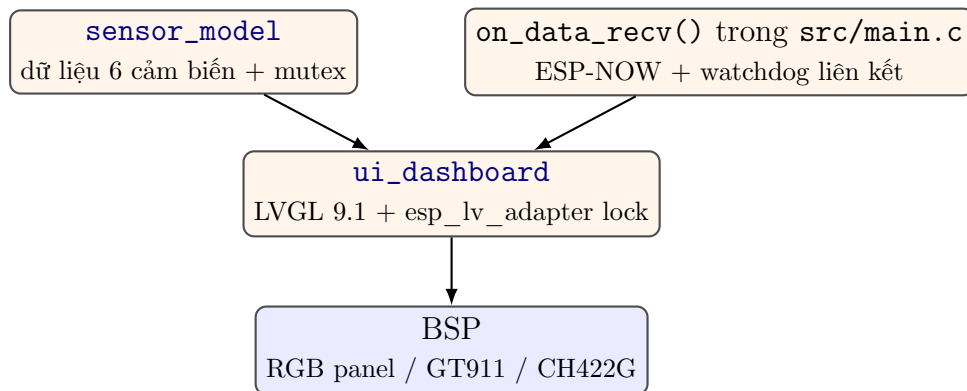
Hình 5: Sơ đồ khối phần mềm của waveshare-screen .
