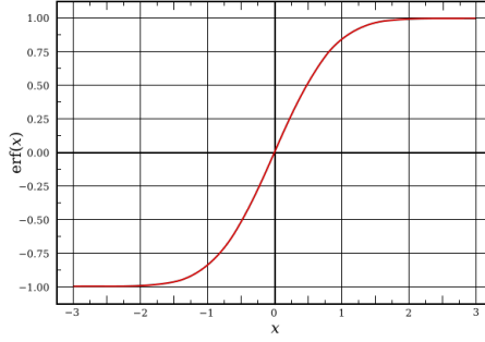
图 12: Error Function
