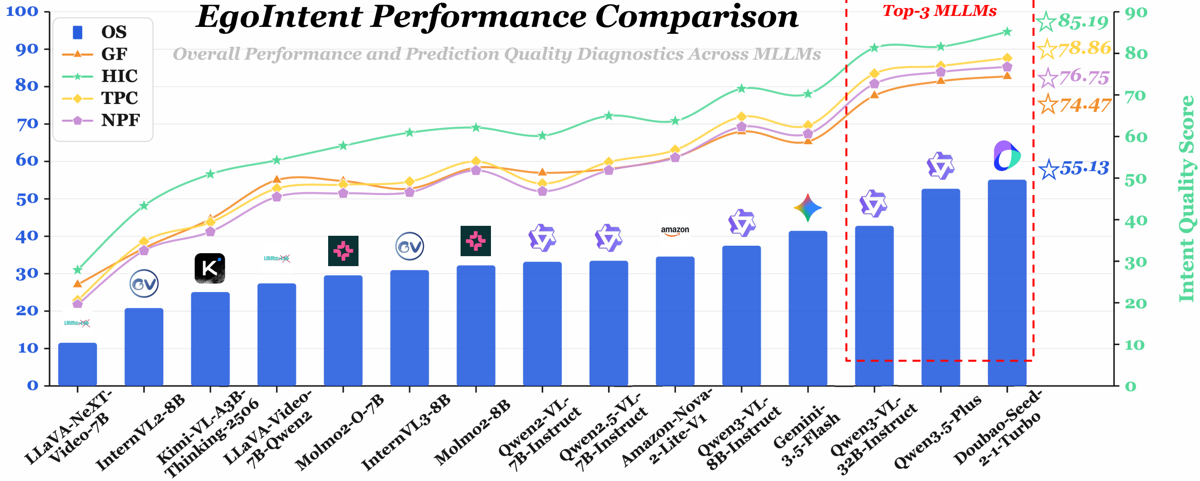
MLLMs Score
