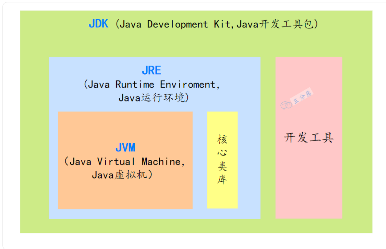
三分恶面渣逆袭：JDK、JRE、JVM关系
