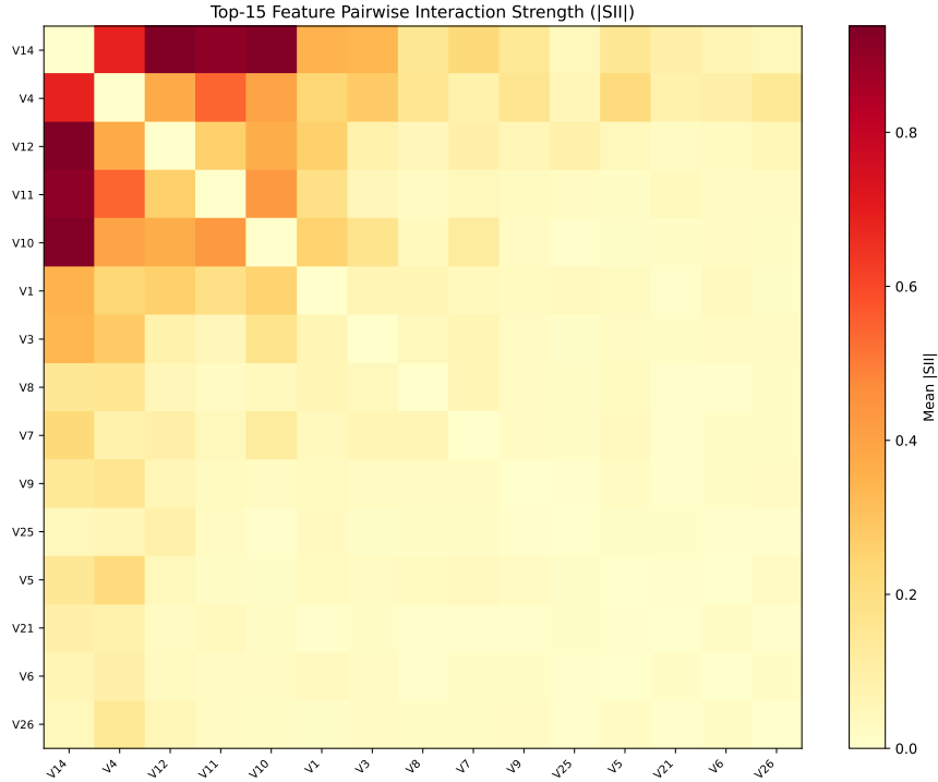
图 12: XGBoost 的 Top-15 特征对 SII 热力图 ( n=50 , shapig TreeSHAP-IQ)。V14 为中心的特征对交互最强。
