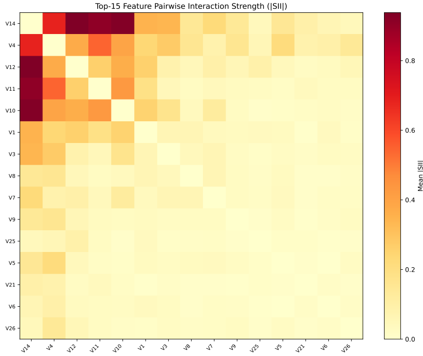
图 12: XGBoost 的 Top-15 特征对 SII 热力图 ( n=50 , shapig TreeSHAP-IQ)。V14 为中心的特征对交互最强。
