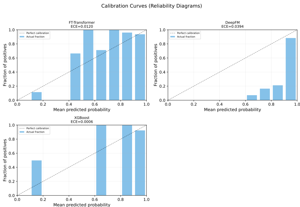
图 13: 各模型的可靠性图。蓝色柱为各概率区间的实际正类率，黑色虚线为完美校准，ECE 标注于子图标题。
