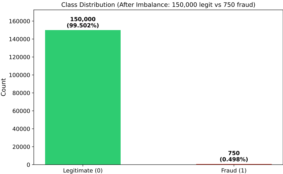
图 1: 经不平衡处理后的数据集类别分布。正常交易 150,000 条，欺诈交易 750 条，正负比约 200:1，准确率在此场景下完全失效。
