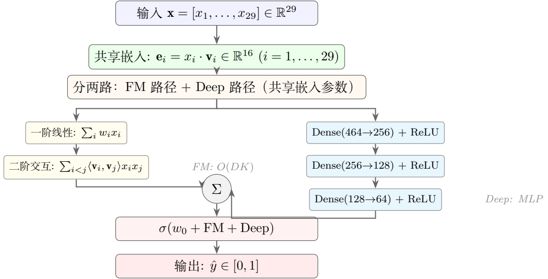
图 4: DeepFM 架构流程图。29 个数值特征经共享嵌入层映射为 16 维向量，分两路并行计算：FM 路径执行显式一阶和二阶特征交互，Deep 路径通过三层 MLP 学习高阶表示。两路输出与全局偏置 w_0 求和后经 Sigmoid 输出。共享嵌入是 DeepFM 的核心设计——FM 的交互质量直接影响 Deep 路径的初始表示。
