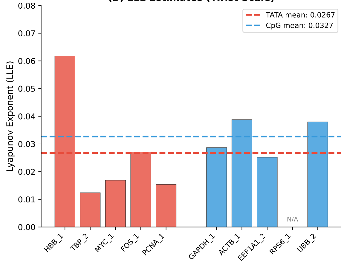
(B) LLE Estimates (Twist Scale)
