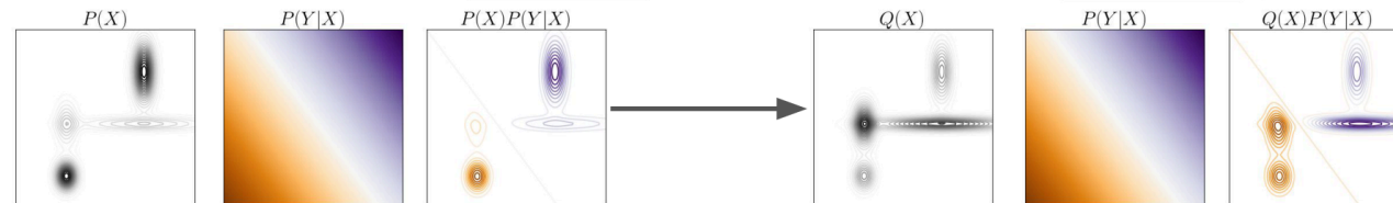
Subpopulation shift
