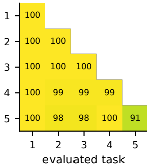
Parameter null
