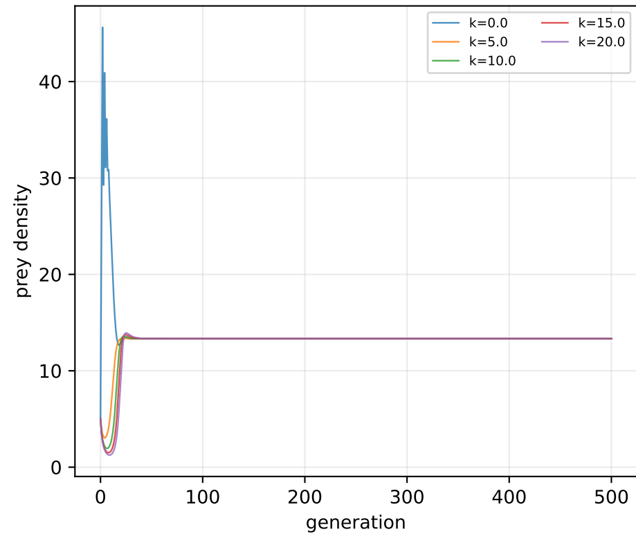
Discrete trajectories
