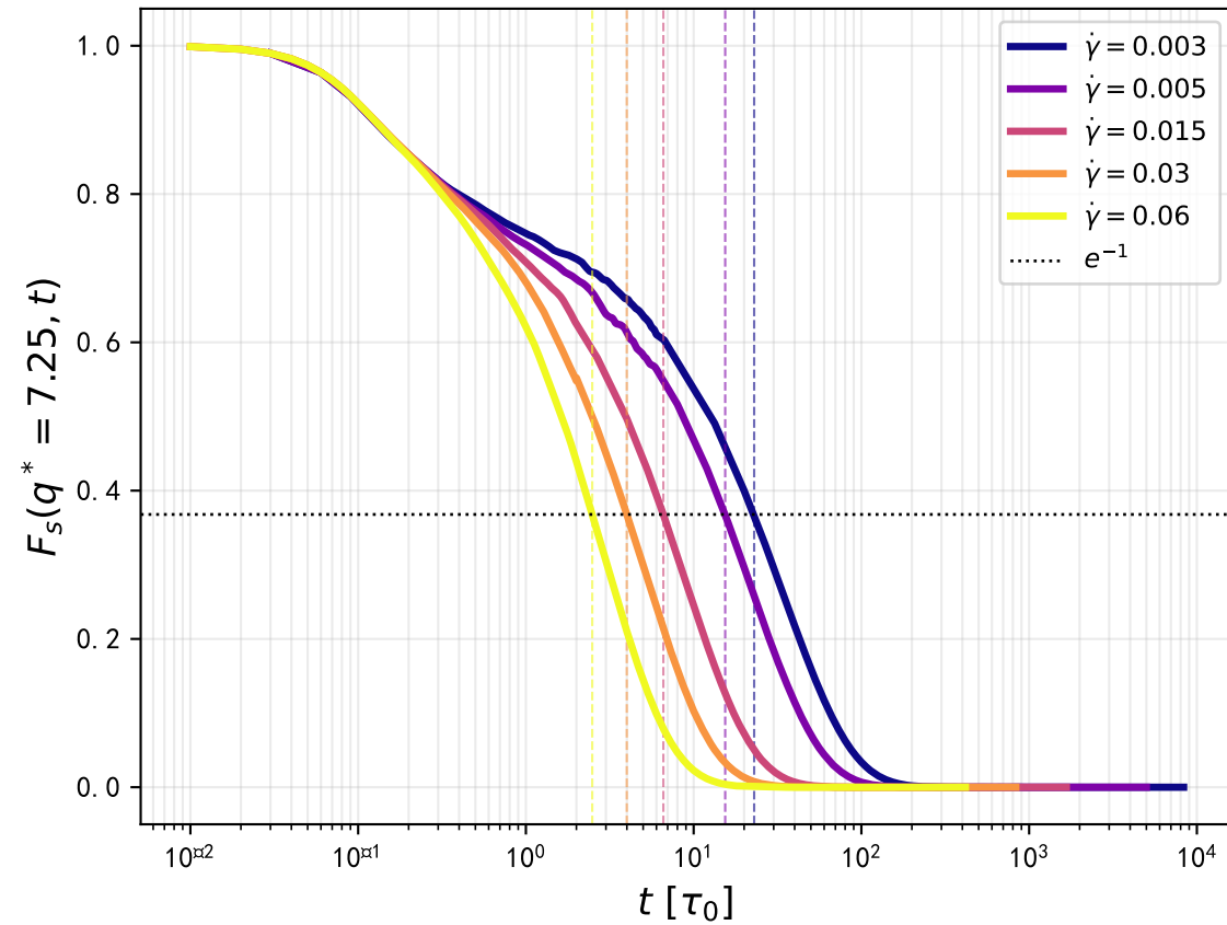
F_s(q^*, t) 各剪切速率对比 T=0.45
