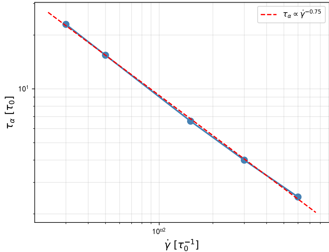
\alpha -弛豫时间 vs 剪切速率
