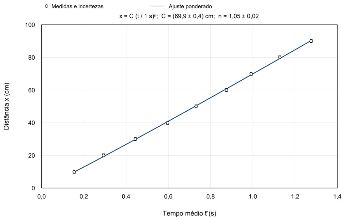
Figura 3 – Lei de potência na escala original
