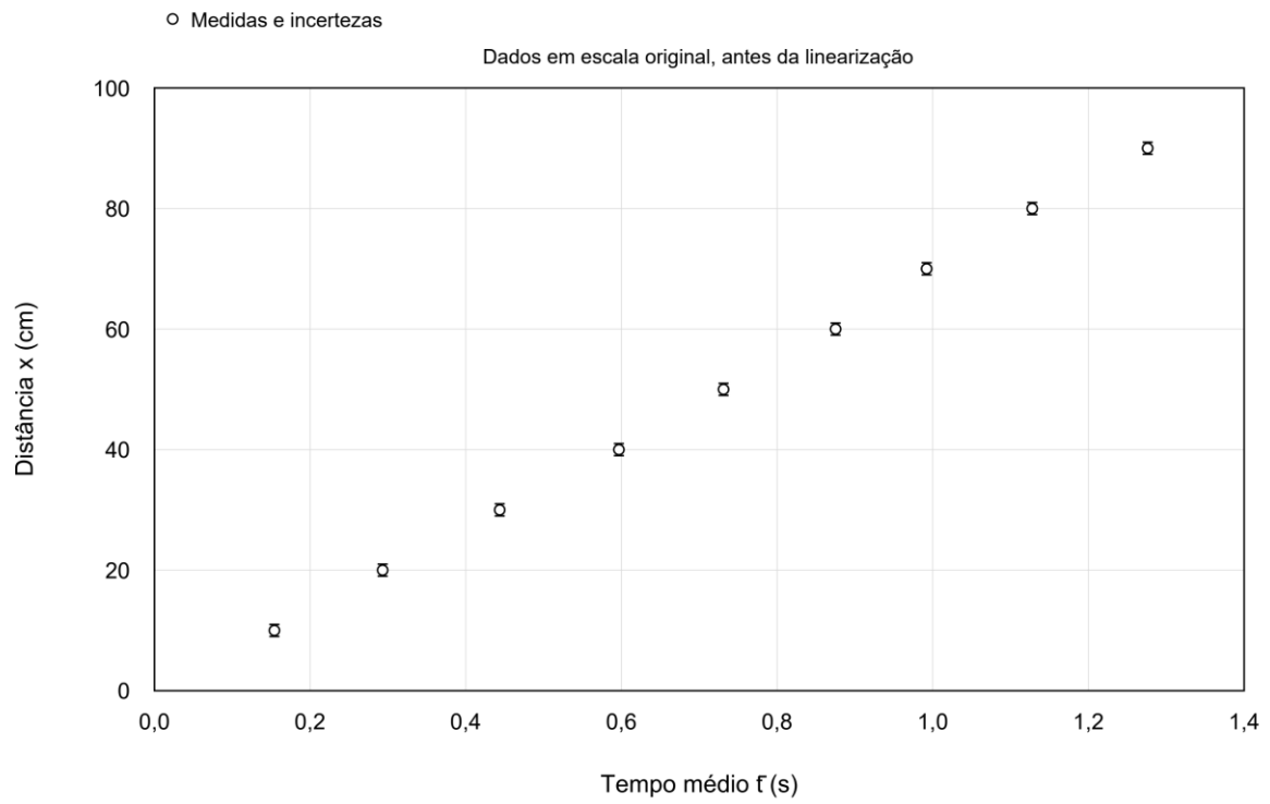
Figura 1 – Dados de distância e tempo antes da linearização
