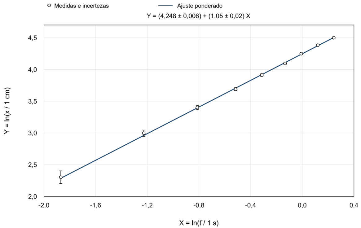
Figura 4 – Linearização logarítmica e reta ajustada
