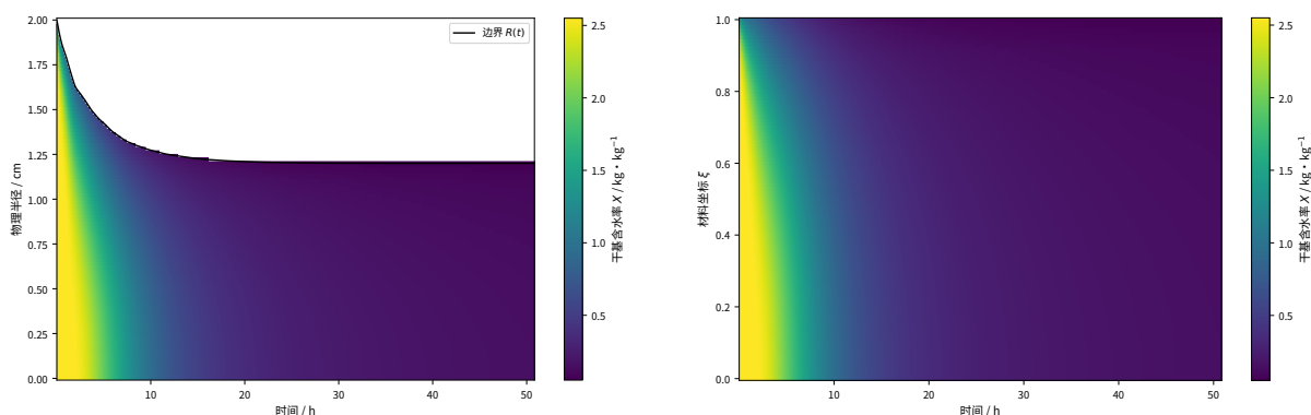
图 6-7 收缩工况含水率场：物理坐标（左）与材料坐标（右）。物理坐标图中的空白区域为收缩后位于药材外部的位罝；两图均由正式 0.1 cm 物理采样结果重构，用于描述宏观分布，不等同于原始 321 单元求解场
