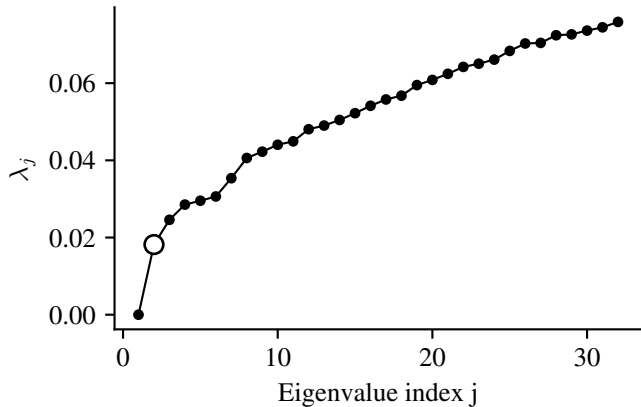
32 smallest eigenvalues
