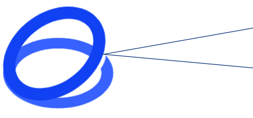
GLM-4.5V-106B
