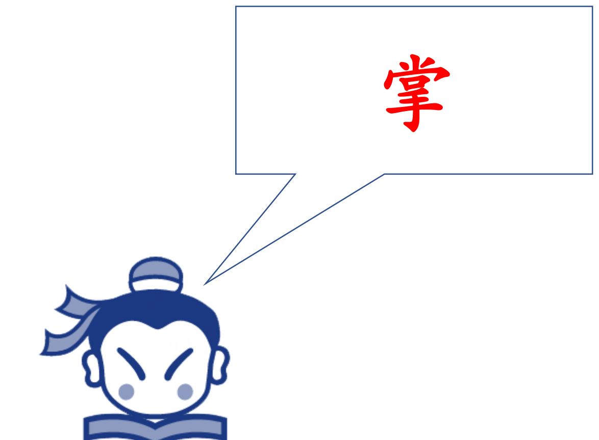
InternVL3.5-1B(LoRA)
