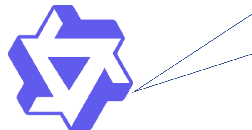
Qwen2.5-VL-3B(SFT)
