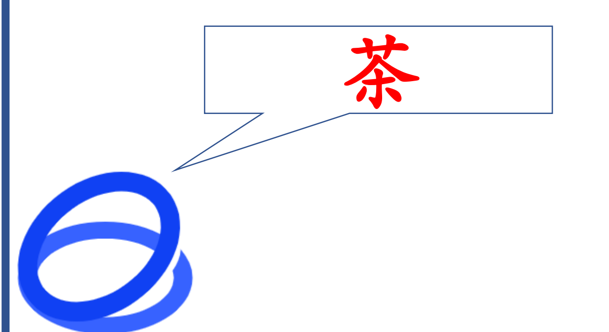
GLM-4.5V-106B
