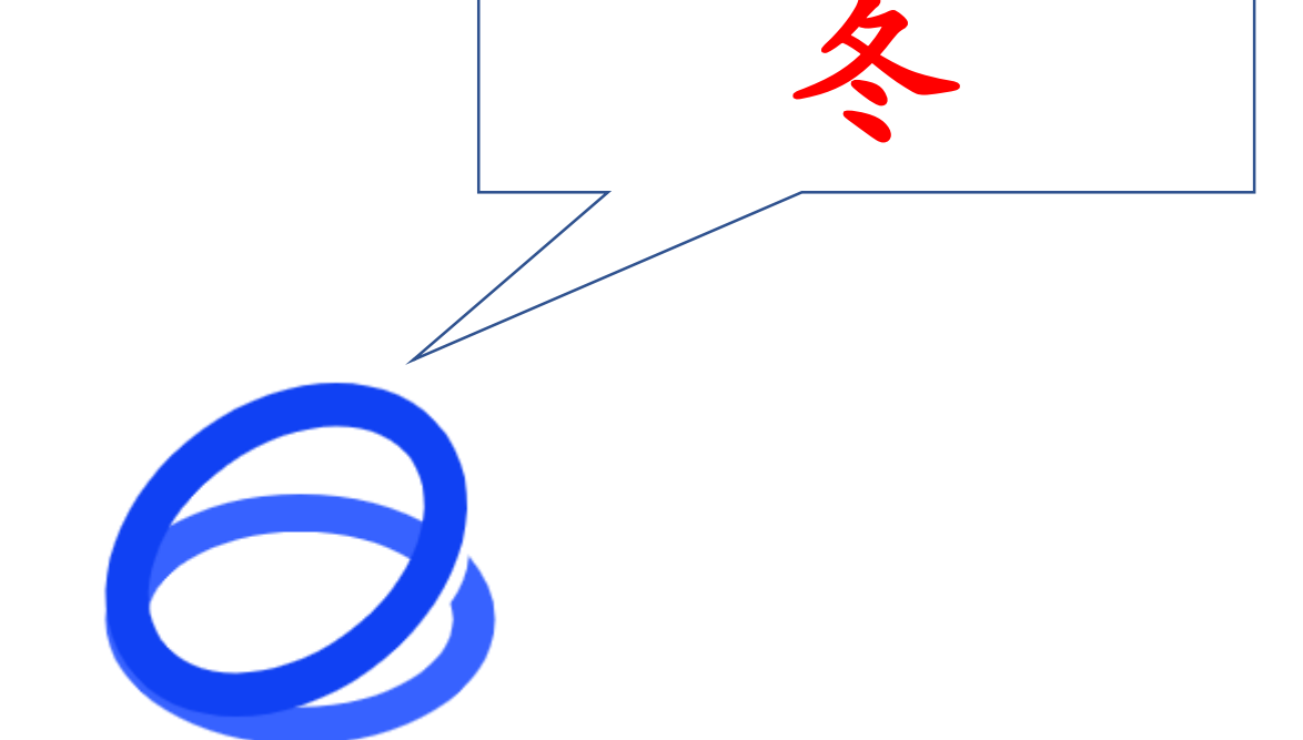
GLM-4.5V-106B
