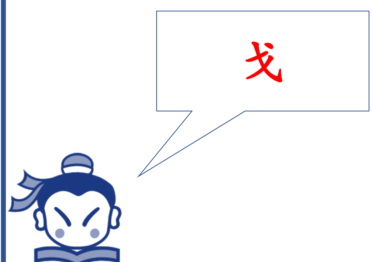
InternVL3.5-1B(LoRA)
