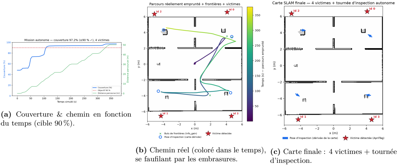
Figure 9: Résultats quantitatifs : 97,17 % de couverture et 4/4 victimes, entièrement autonome. La trajectoire est le chemin réel dans le repère carte ; les murs sont dessinés par-dessus, si bien qu'elle passe visiblement par les embrasures (vérifié : aucun segment ne traverse un mur).
