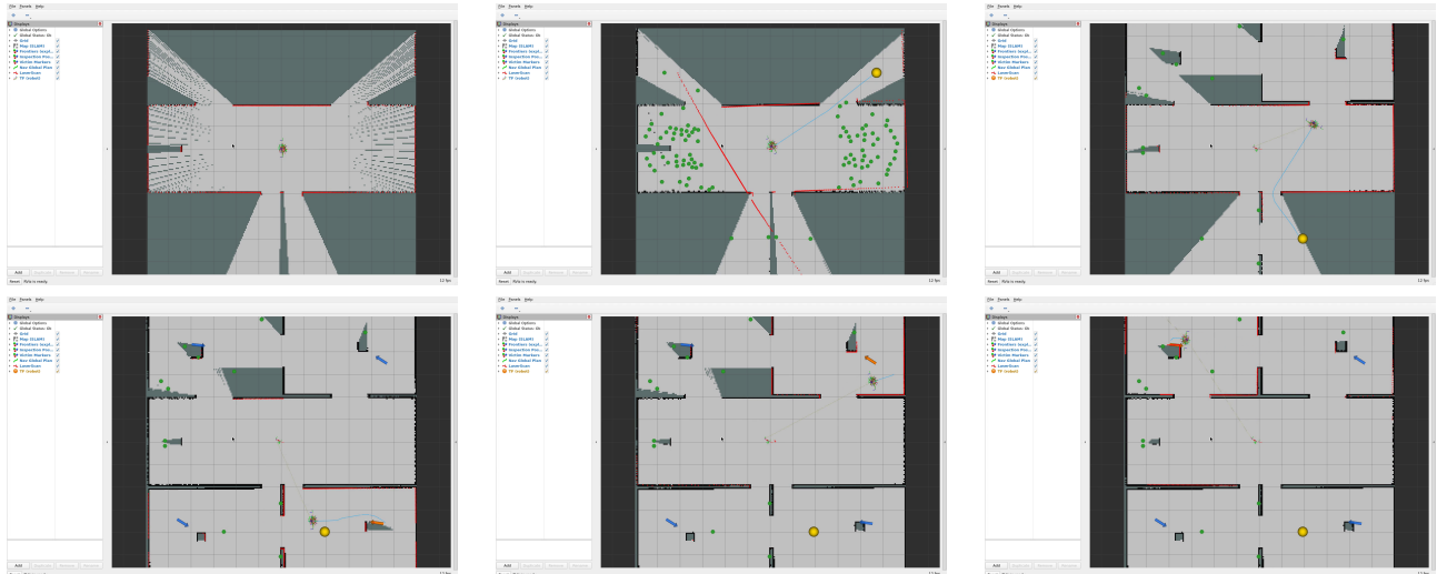
Figure 8: RViz en direct à six moments clés (1–3 : exploration précoce, carte presque construite, transition de phase ; 4–6 : inspection des pièces, victimes apparaissant, carte finale) - montrant la carte (SLAM), les frontières, les poses d'inspection, le plan Nav2, le LaserScan et les quatre marqueurs de victimes. Capturé en HD sur un serveur X virtuel.
