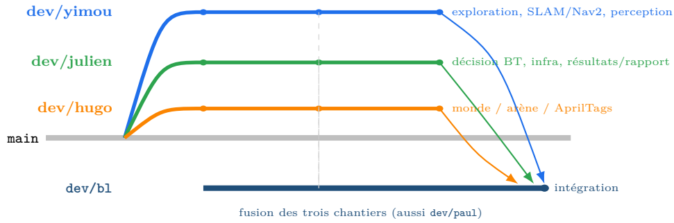
Figure 7: Construction des branches : trois branches de fonctionnalités par développeur (chantiers issus de l'historique git) sont fusionnées dans dev/bl , la branche d'intégration.
