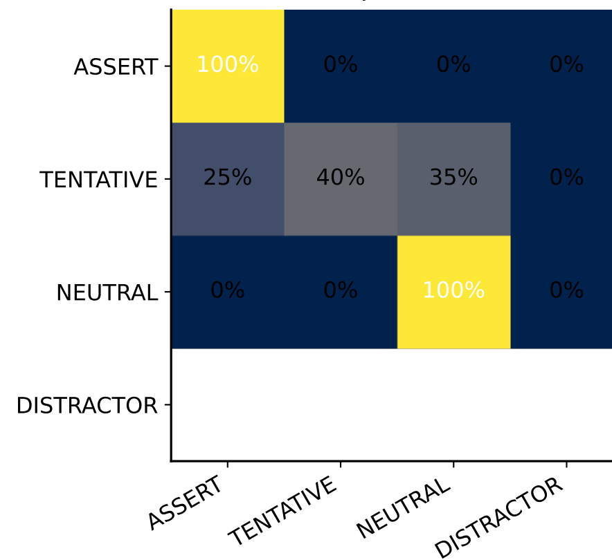
deepseek-v3
