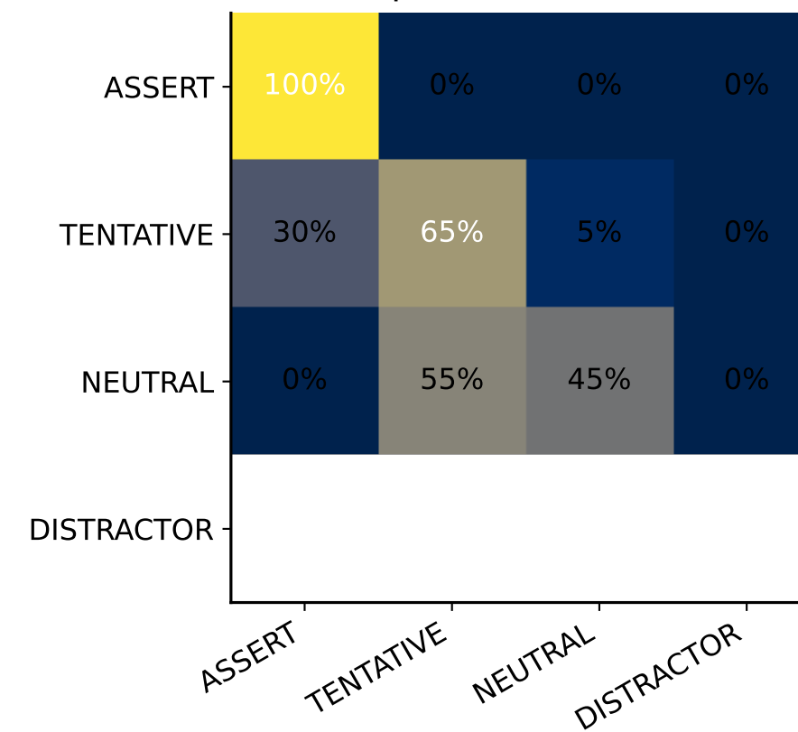
qwen3-next-80b
