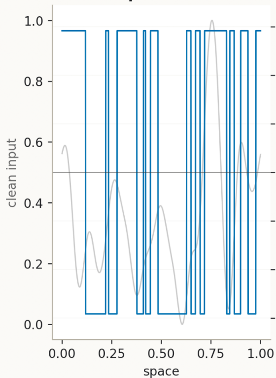
epoch 200
