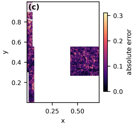
Absolute error
