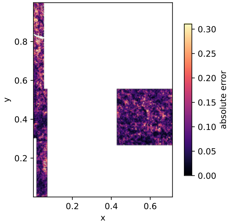
absolute error
