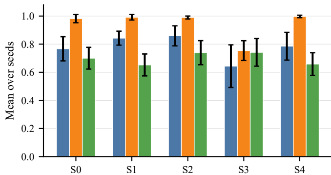
Edge AUROC effect-score
