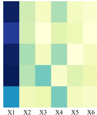
TE
