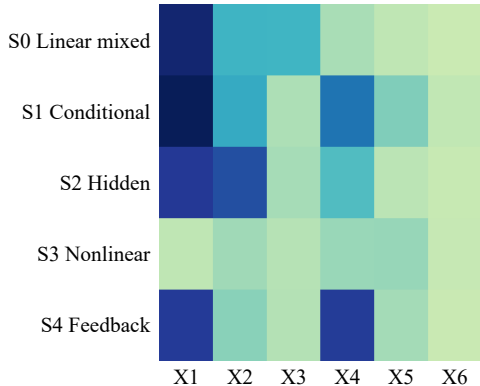
VAR-GC
