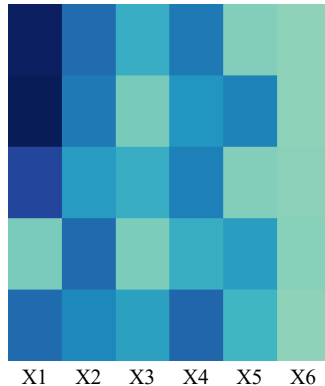
PCMCI-ParCorr
