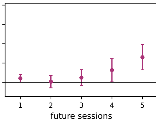
Zhou2020
