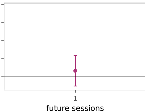
Zhou2016
