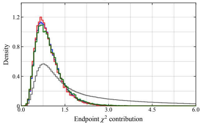
A. Endpoint \chi^2
