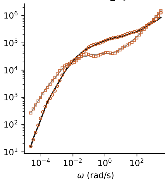
(d) M1 T=150°C rel_log=0.044
