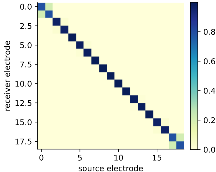
Spatial diffusion kernel K
