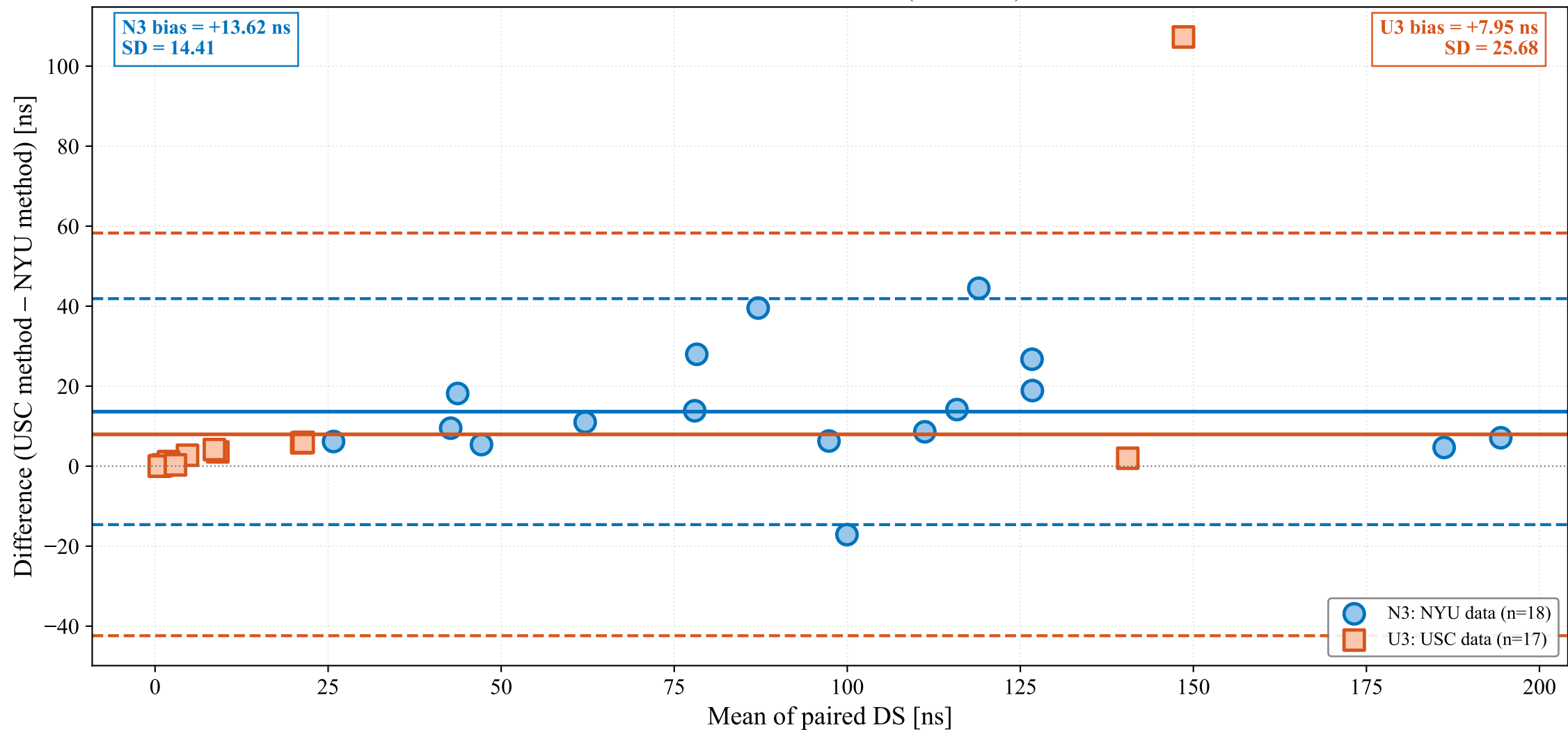
Bland-Altman: Omni DS (6.75 GHz)
