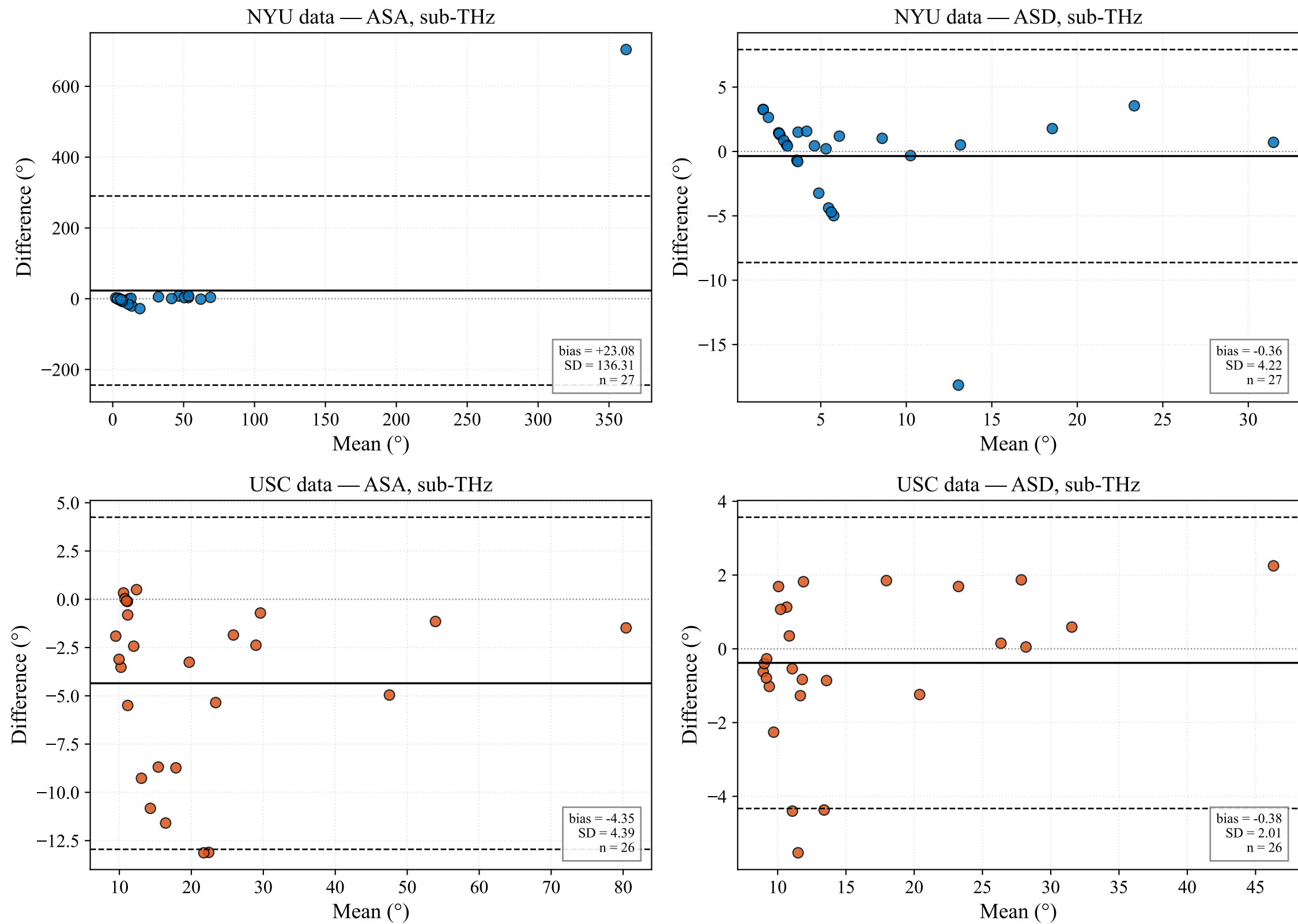
Fig. 4 — Bland-Altman: ASA & ASD cross-processing (sub-THz)
