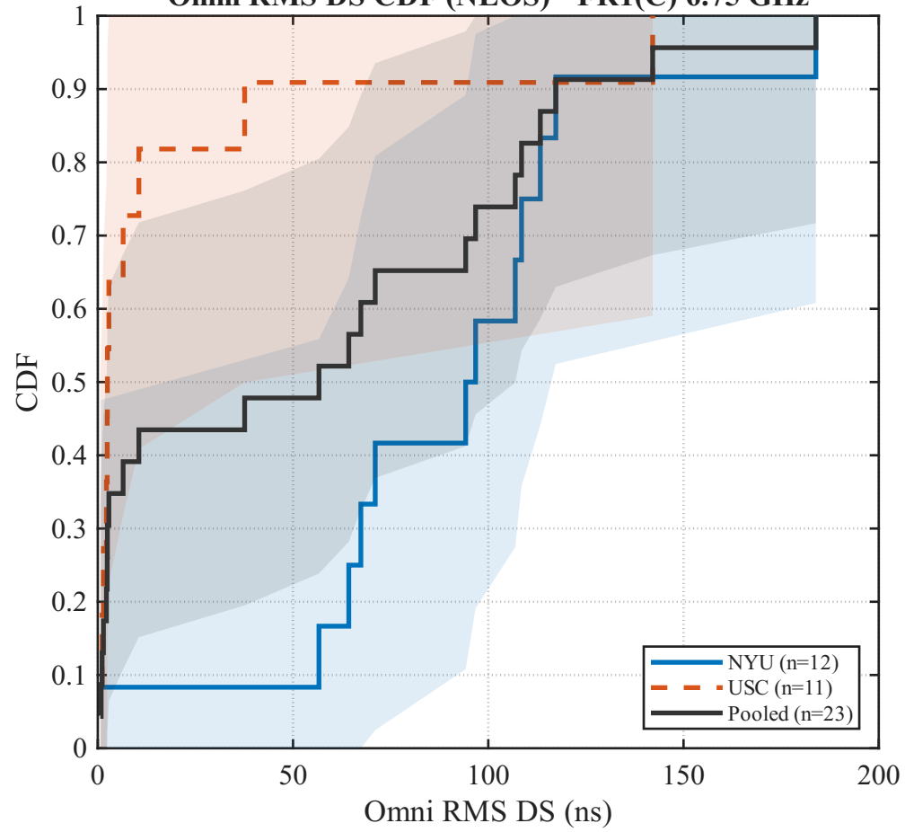
Omni RMS DS CDF (NLOS) - FR1(C) 6.75 GHz
