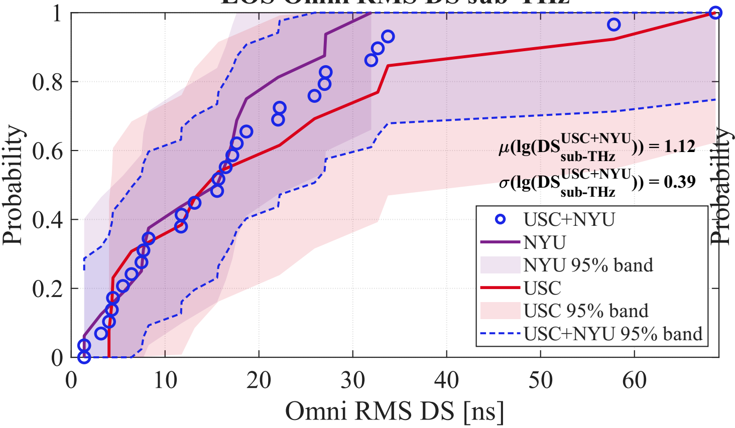
LOS Omni RMS DS sub-THz
