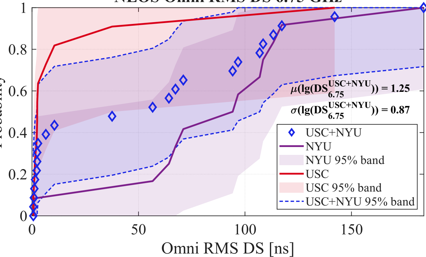
NLOS Omni RMS DS 6.75 GHz
