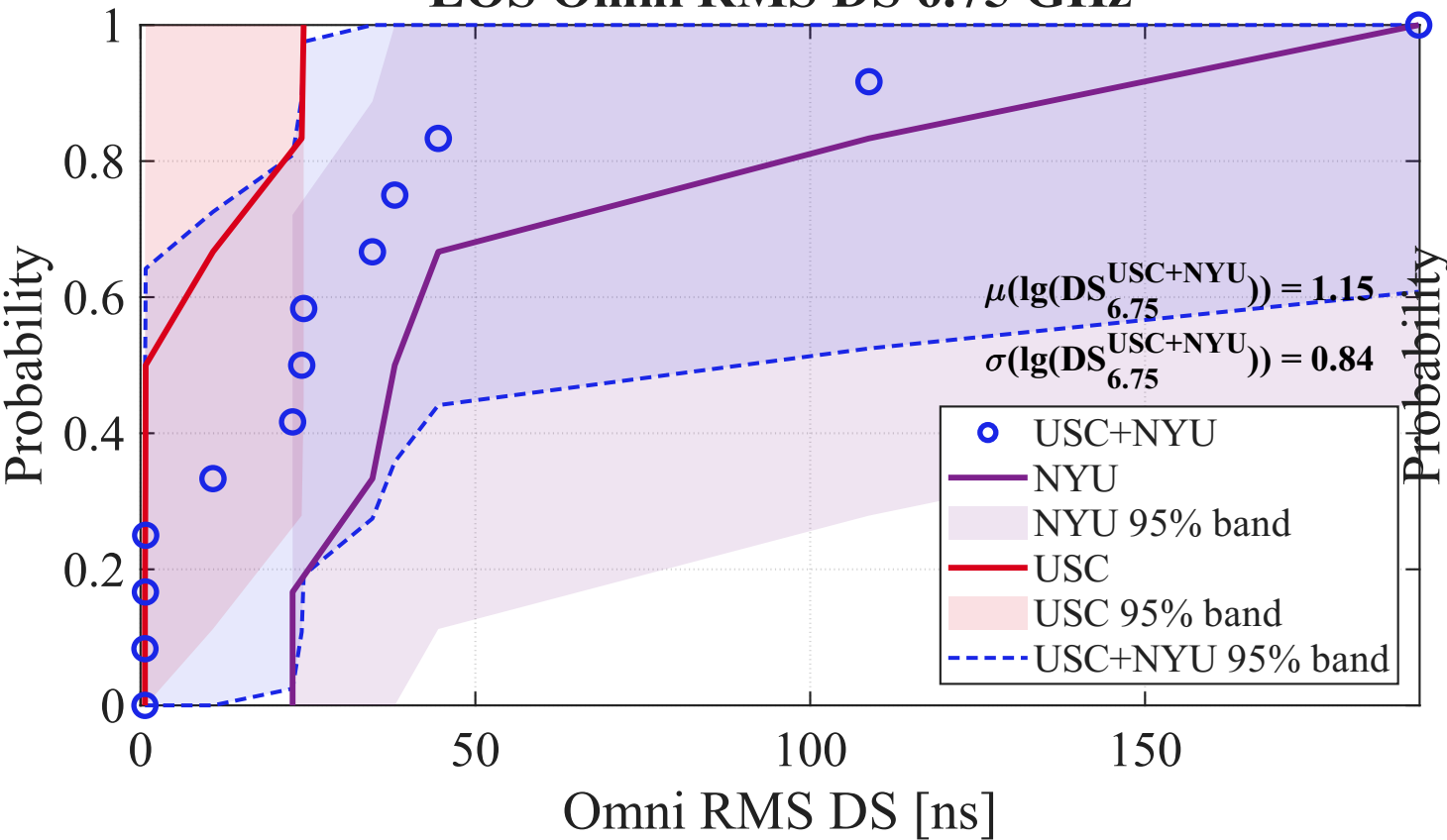
LOS Omni RMS DS 6.75 GHz
