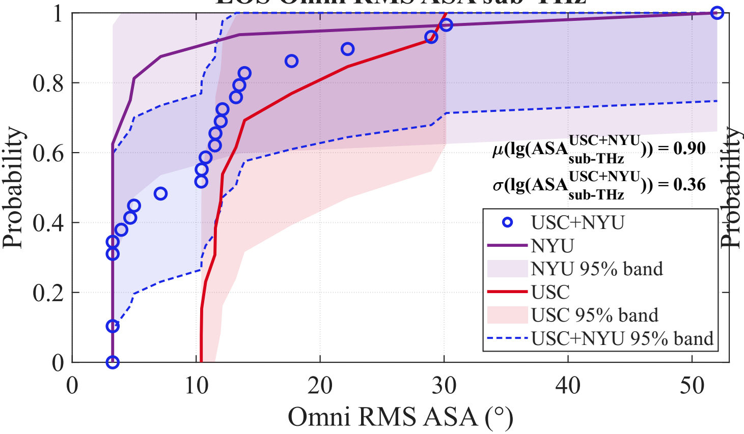
LOS Omni RMS ASA sub-THz
