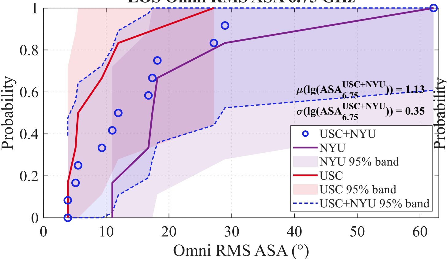
LOS Omni RMS ASA 6.75 GHz
