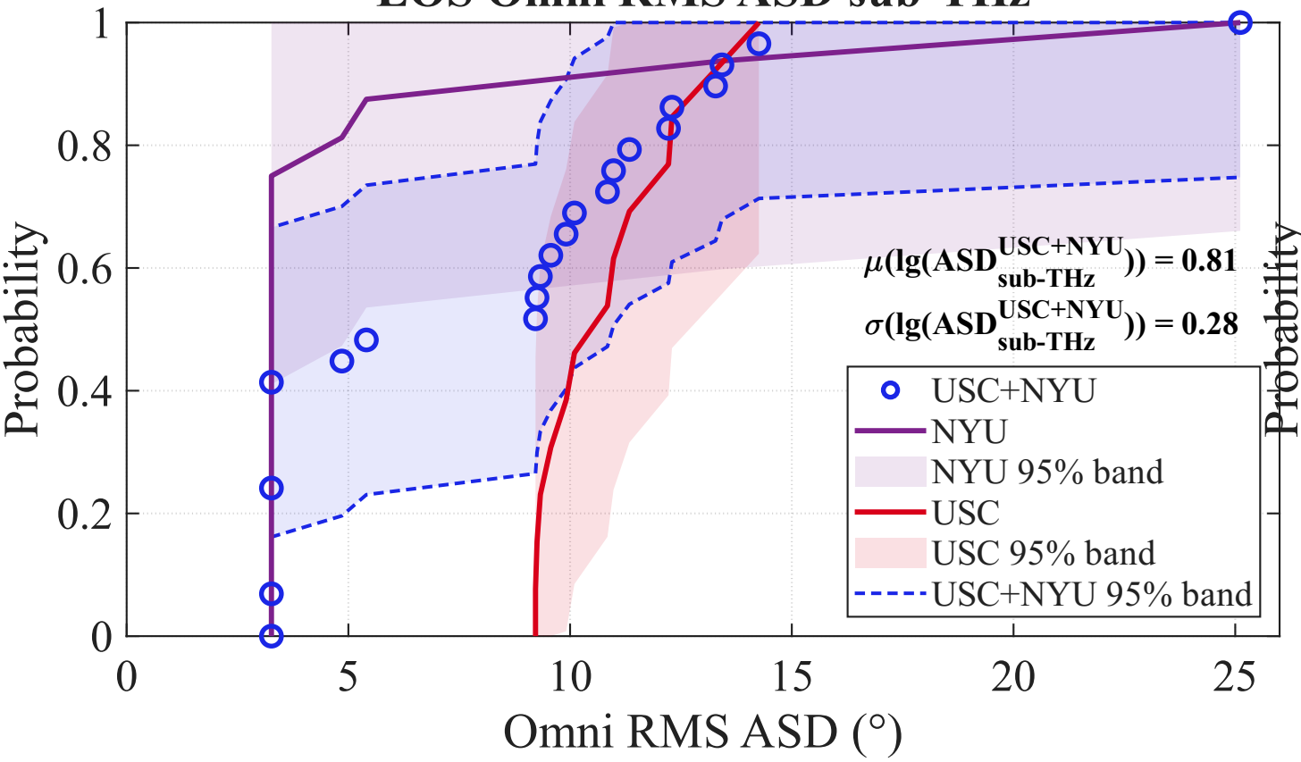
LOS Omni RMS ASD sub-THz
